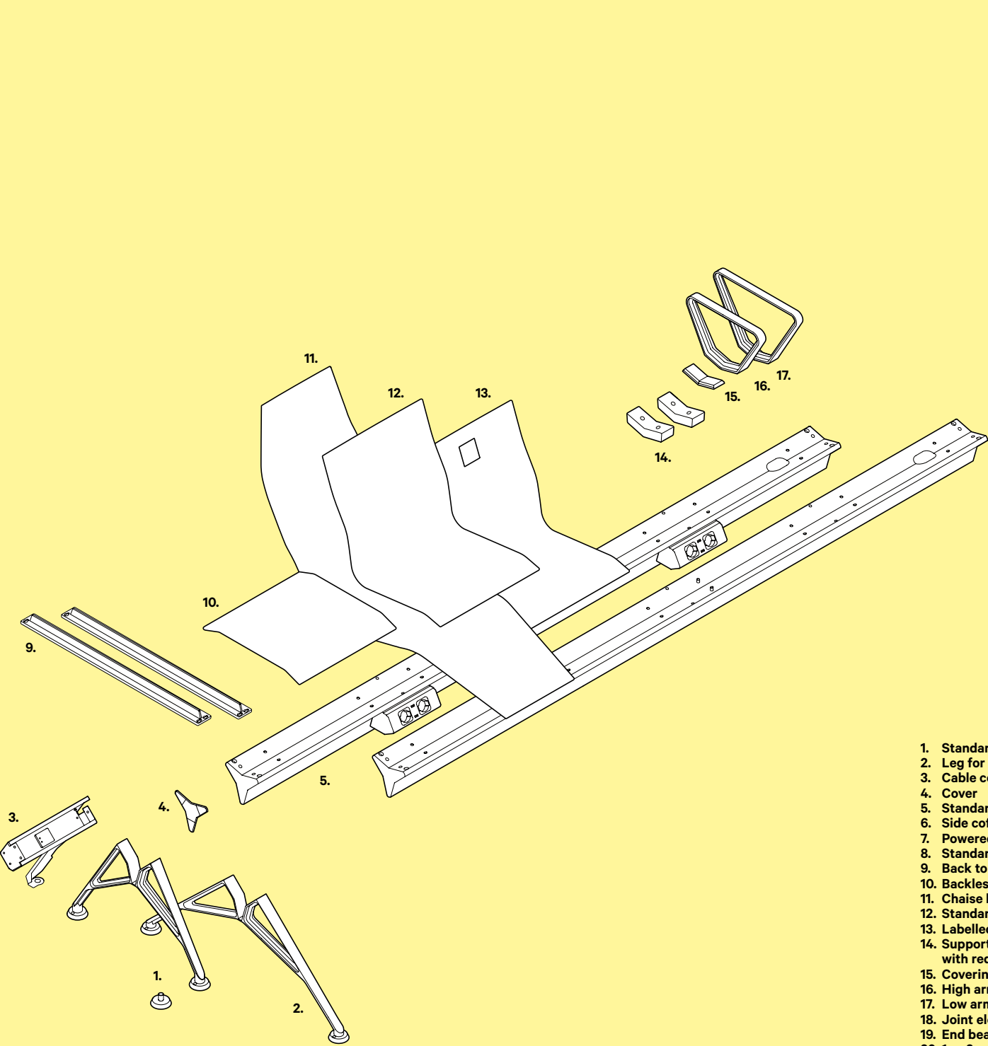
Exploded view of all Aeris seating system elements. Esploso dei componenti del sistema Aeris.
